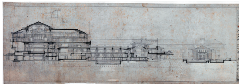
帝国ホテル二代目本館 第2案 縦断面図 コロンビア大学エイヴリー建築美術図書館 フランク・ロイド・ライト財団アーカイヴズ蔵
