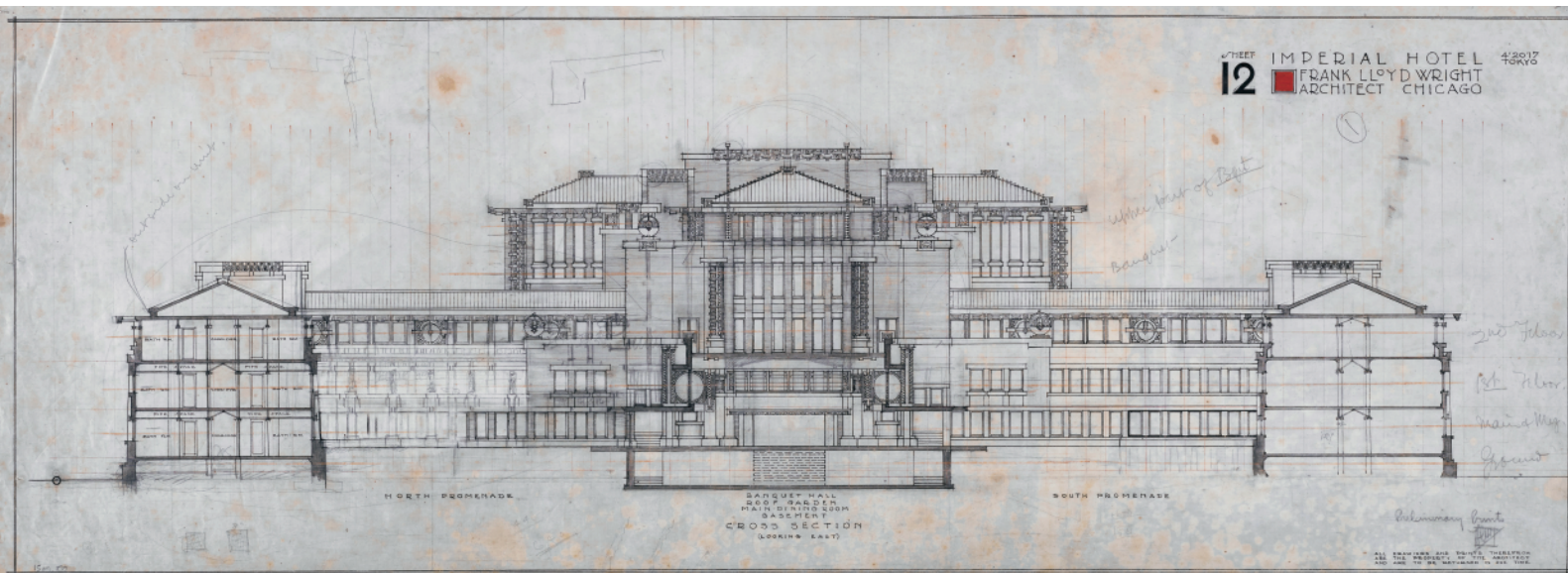
帝国ホテル二代目本館 第2案 横断面図
